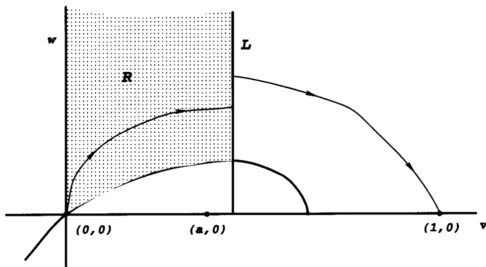
The region R
