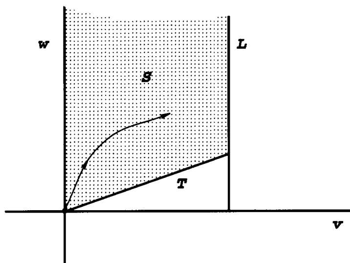
The region S
